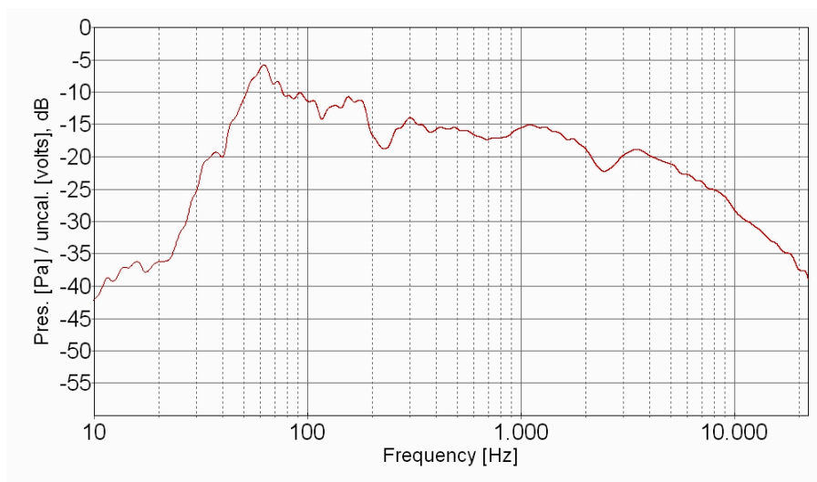
Σχήμα 5: Απόκριση συχνότητας αίθουσας με εξομάλυνση 1/6 οκτάβας
